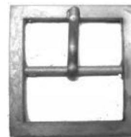
HJB-008, 1-1/8"X1-1/8"日字针扣, 单重: 10.414g
